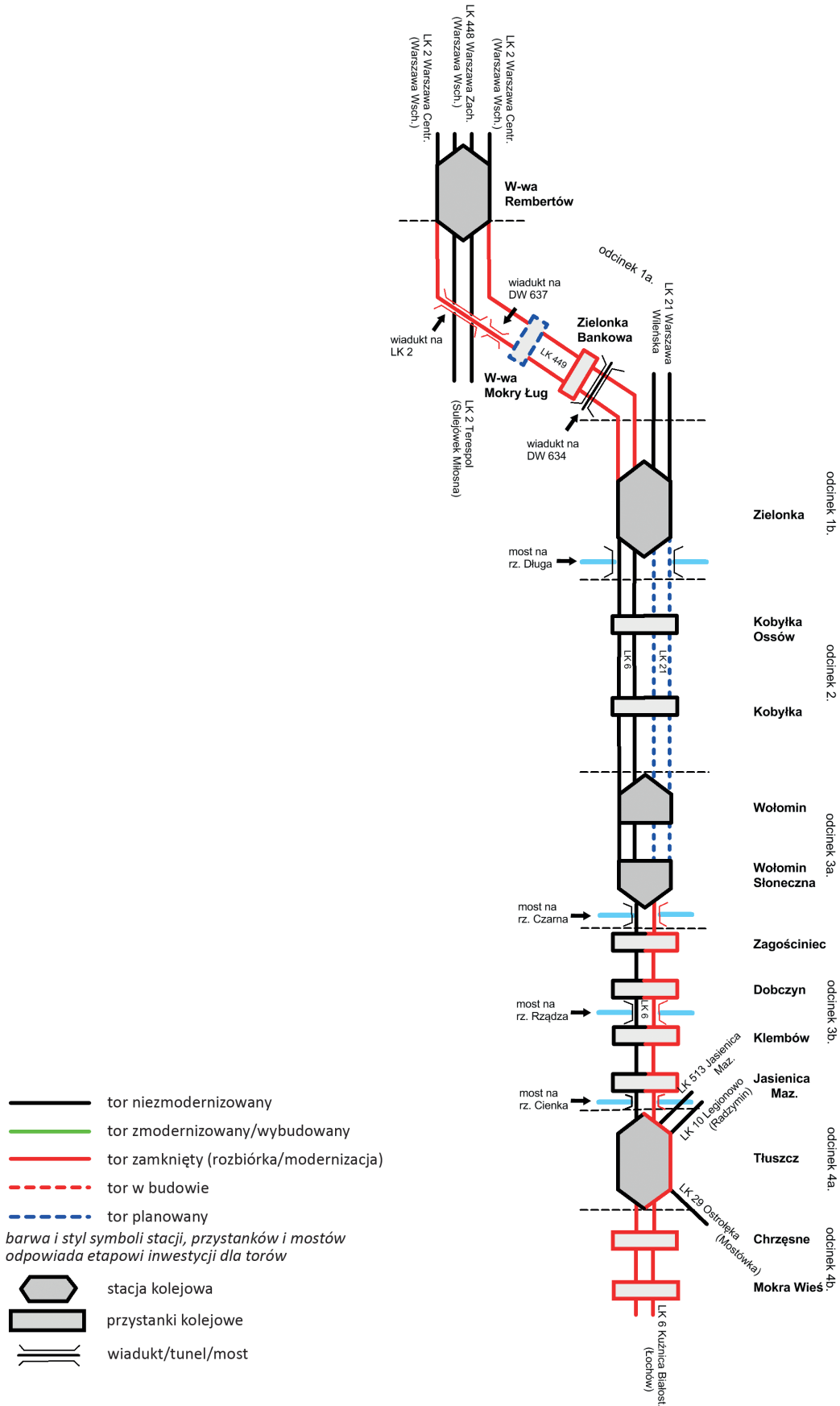
Ryc. 51. Stan modernizacji linii kolejowej E75 na koniec 2014 r. Źródło: opracowanie MBPR
